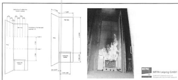
図18 BS8414-1による外壁火災試験
