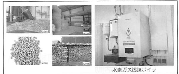
図4 バイオマスと水素エネルギー暖房の設置
