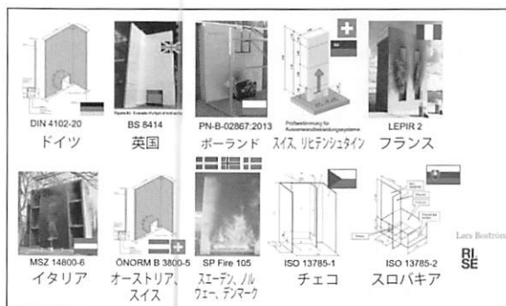
図16 欧州での現状の火災試験方法
